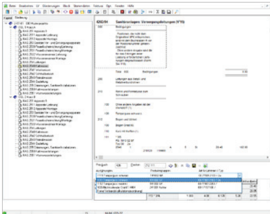
Finestra di dialogo per il rilevamento secondo OGL/KAG
