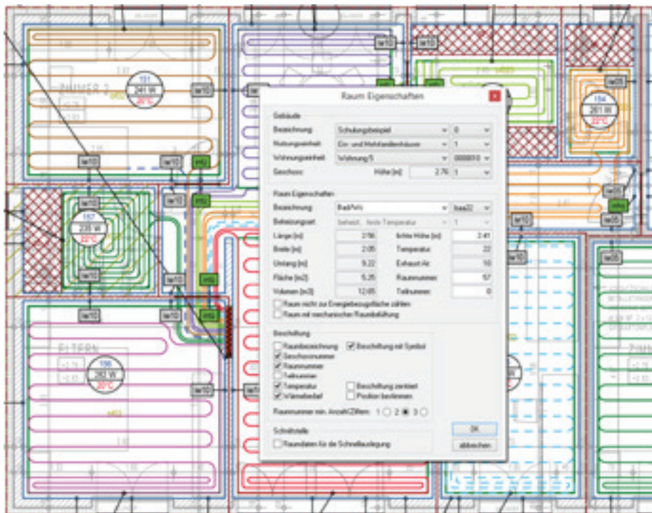
Plan de pose du chauffage par le sol avec les données techniques de Win_HT pro
