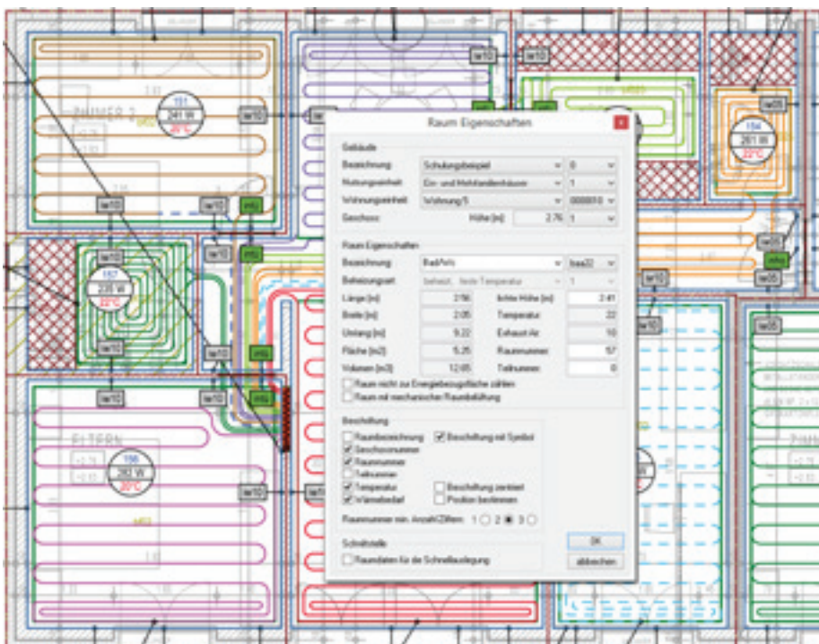
Progetto di posa del riscaldamento a pavimento con i dati tecnici di Win_HT pro
